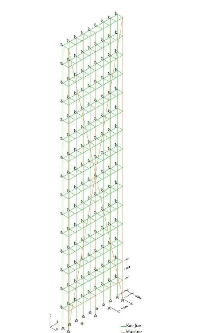
Fig.5 Schema statico di un'impalcatura di bambù
