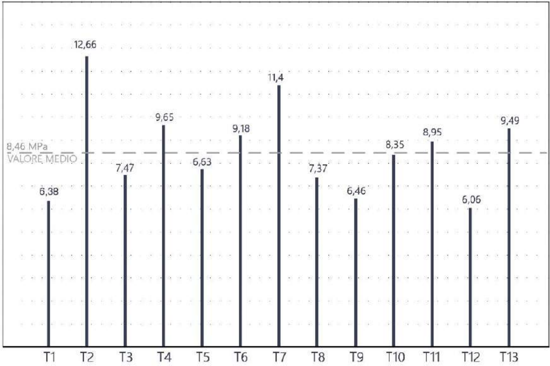
Fig.8 I valori della resistenza a taglio
