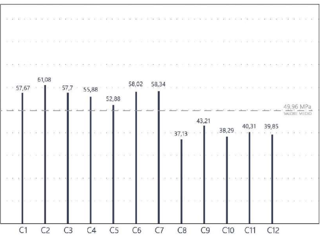
Fig.7 I valori della resistenza a compressione
